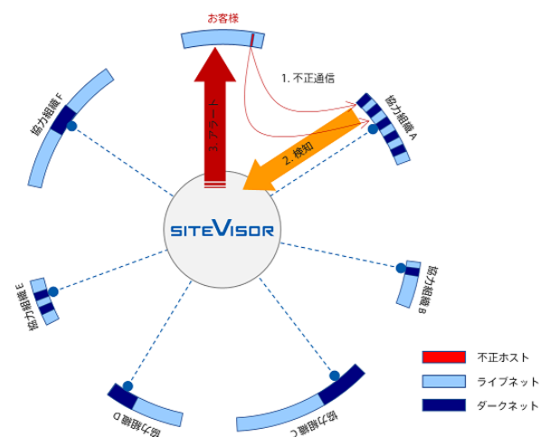
SiteVisor が不正通信を検知する仕組み
